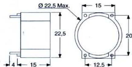
2 : Boîtier Horizontal / Horizontal case
