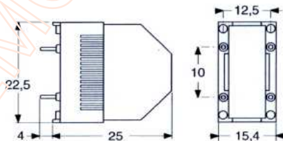
1 : Boîtier Vertical / Vertical case
